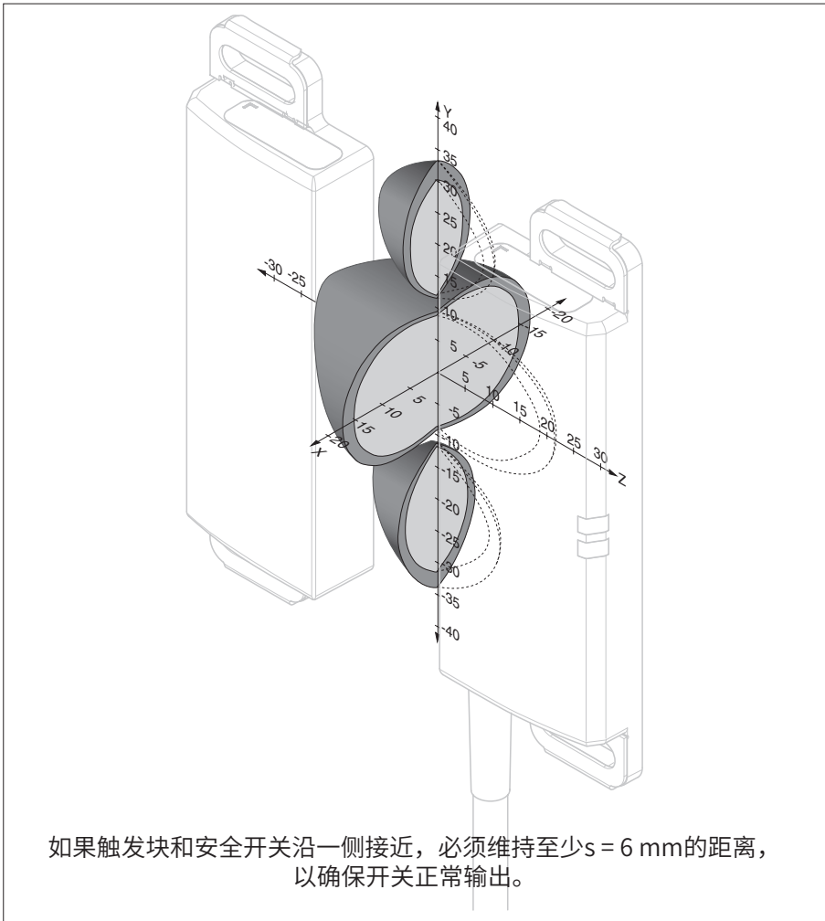
图6：典型工作距离
