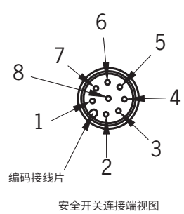
图2：CES-AR安全开关的接头分配
