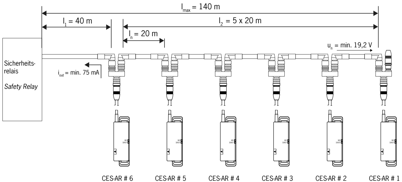
图1：带六个CES-AR安全开关的电路示例
