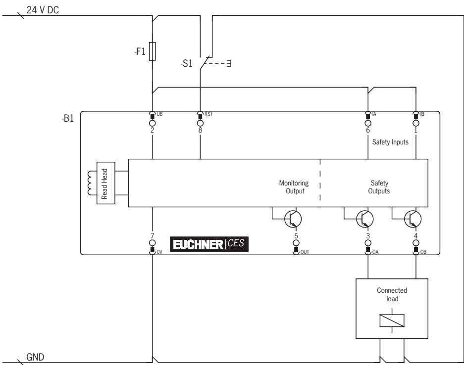
图3：CES-AR-...单独工作的接配线示例
