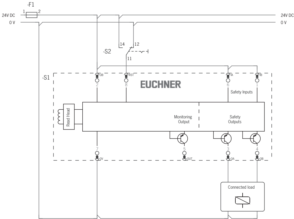
图3：CES-AR-...单独工作的接配线示例
