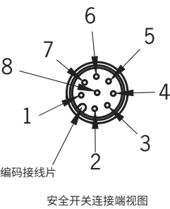
图2：CES-AR-C01安全开关的接头分配
