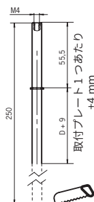
延長アクチュ エーション軸
