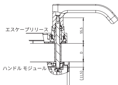
取付プレートなしの例
