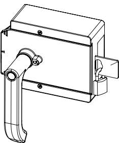
図 1: 南京錠で固定されたロックアウト機構
