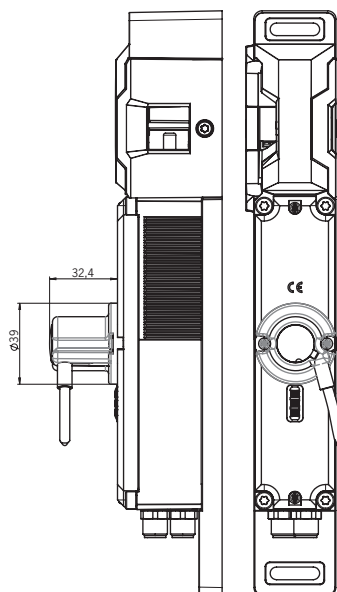
ワイヤ・フロント・リリース (ボーデン) を装着
