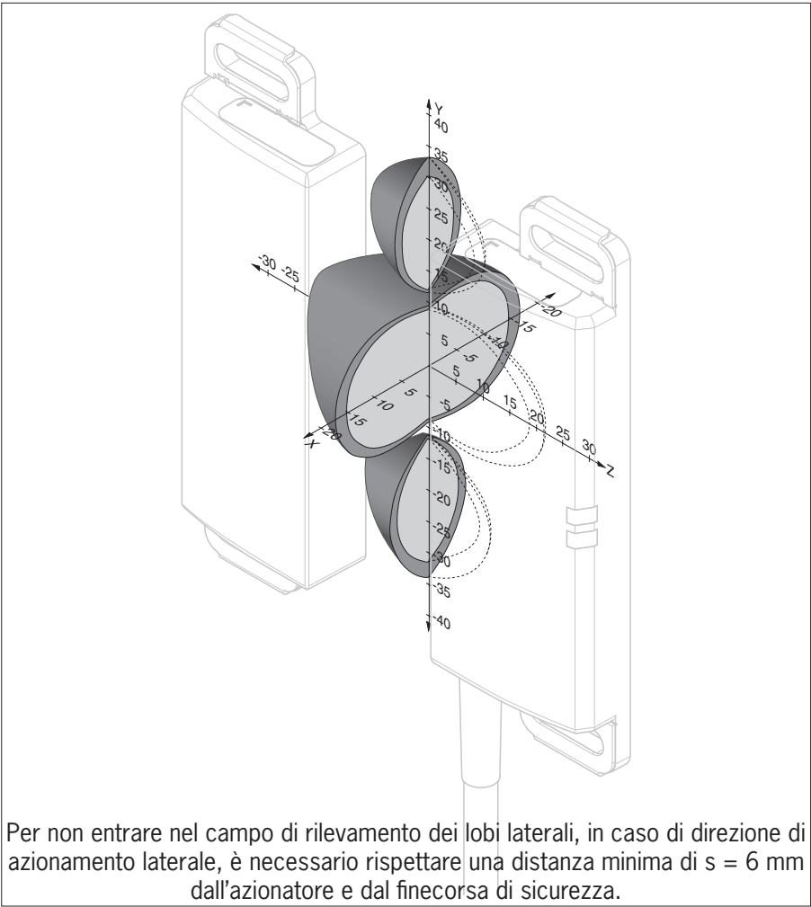
Fig. 4: Campo di rilevamento tipico
