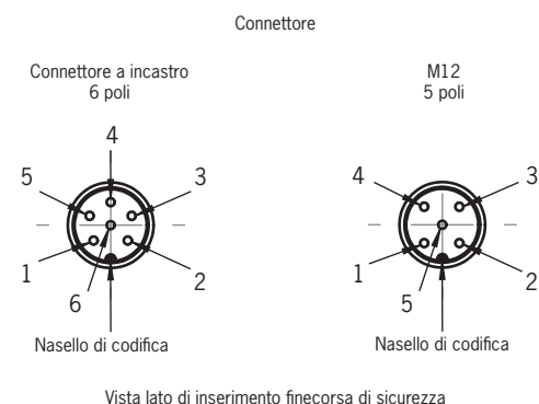
Fig. 1: Collegamenti finecorsa di sicurezza CES-AP-C.2
