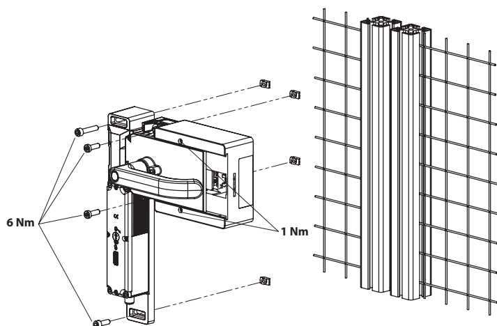
Fig. 2 : Situation de montage sans déverrouillage interne
