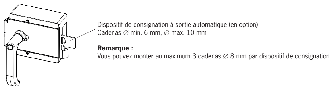
Fig. 1 : Dispositif de consignation verrouillé par un cadenas
