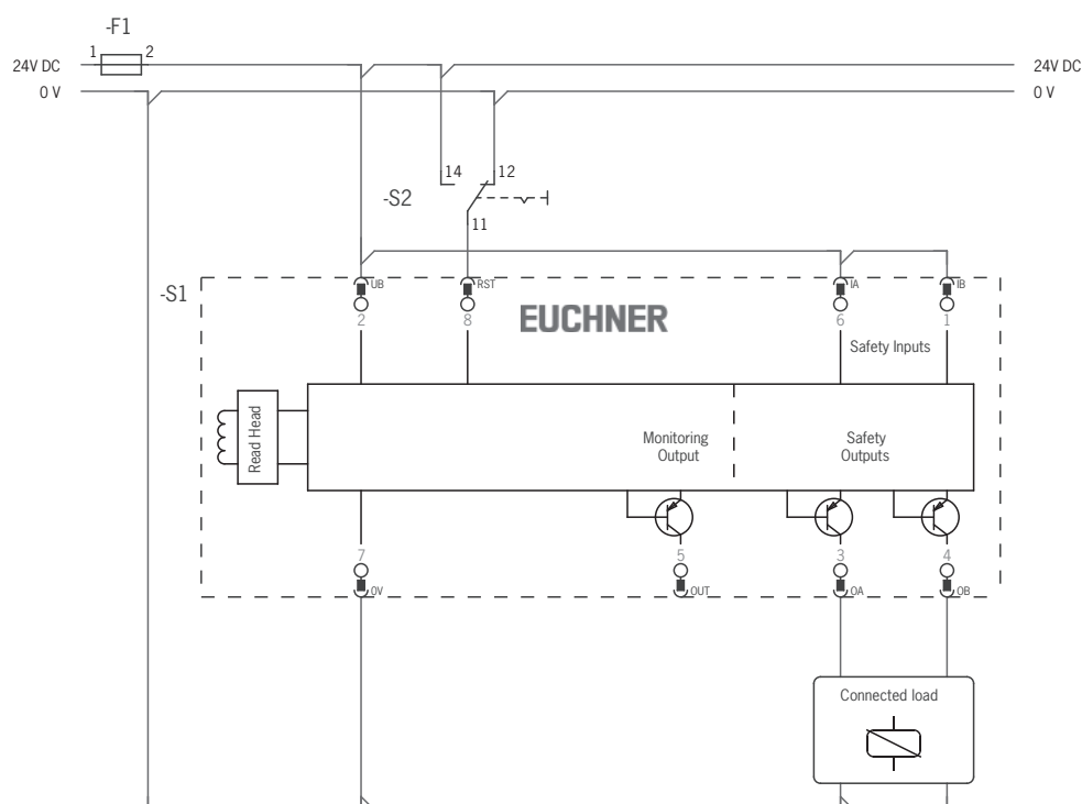
Fig. 3 : Exemple de raccordement interrupteur individuel CES-AR...
