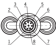
Distribuidor en Y con cable de conexión 111696 o 112395
