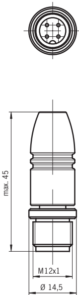
Conector puente 097645 4 polos, macho (fig. similar)
