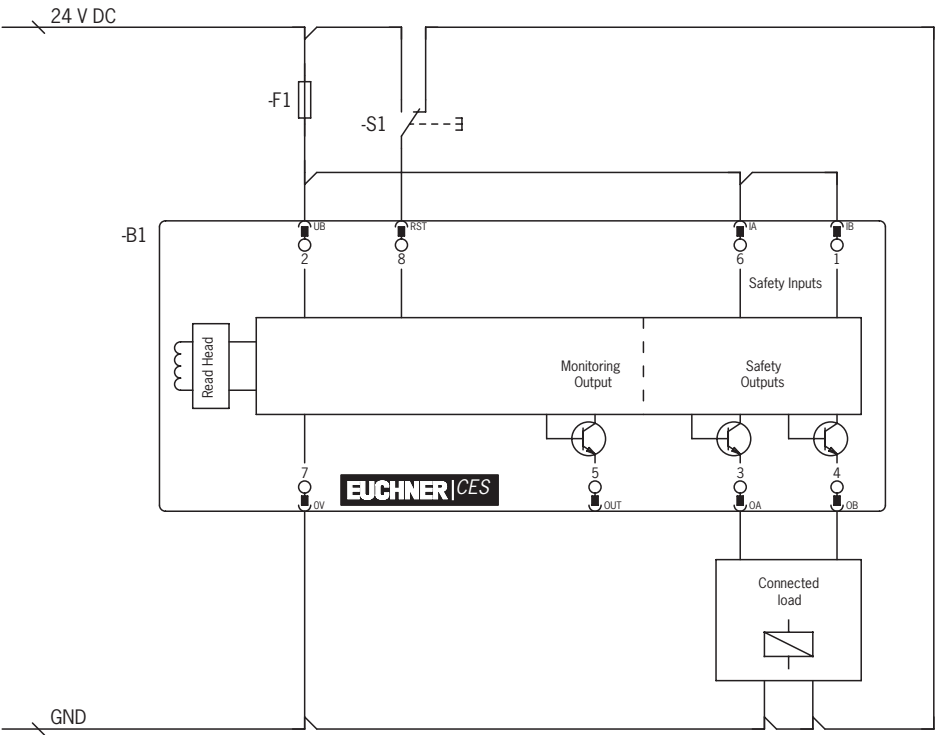
Fig. 3: Ejemplo de conexión para funcionamiento independiente de un dispositivo CES-AR...
