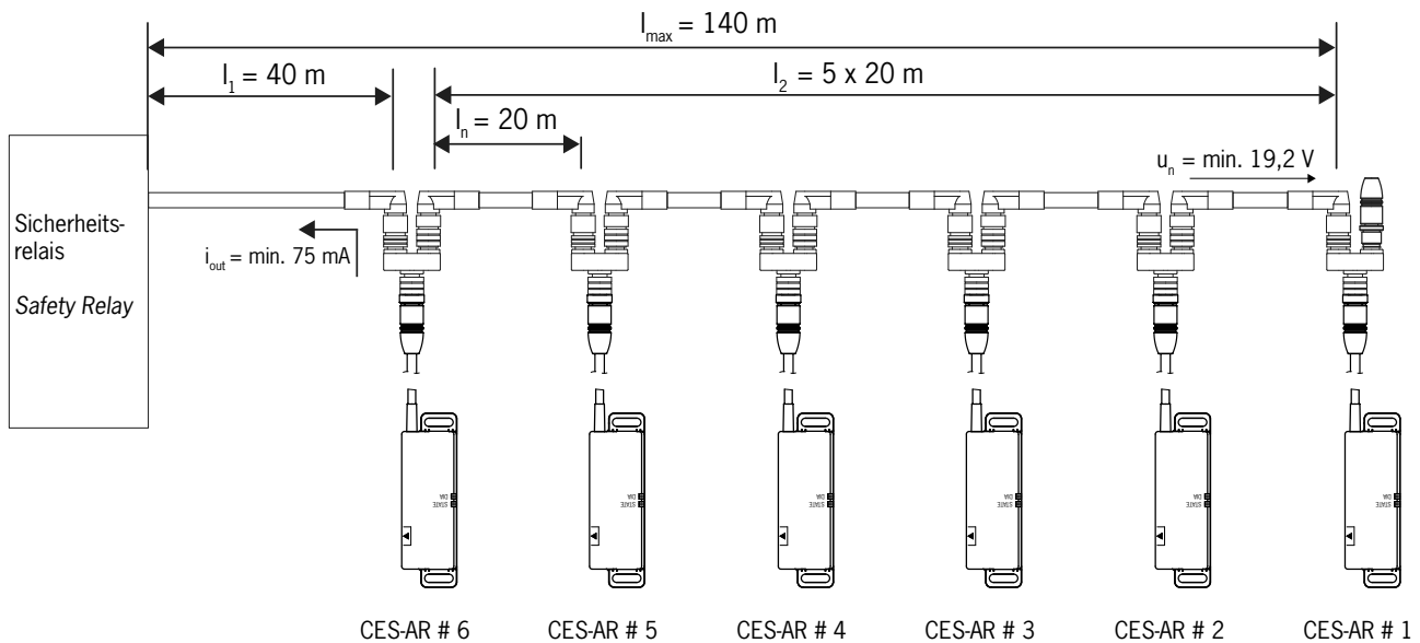
Fig. 1: Ejemplo de conexión de seis interruptores CES-AR
