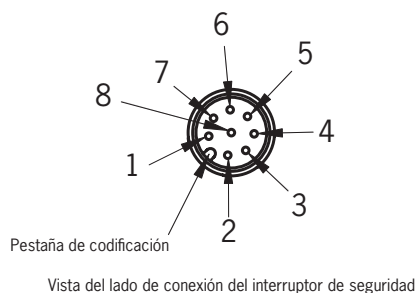
Fig. 2: Asignación de contactos del interruptor de seguridad CESAR
