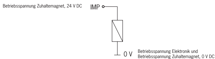
Bild 7: Anschlussbeispiel ohne Anschluss IMM
