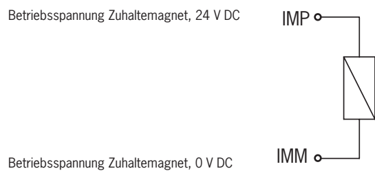
Bild 6: Anschlussbeispiel mit Anschluss IMM
