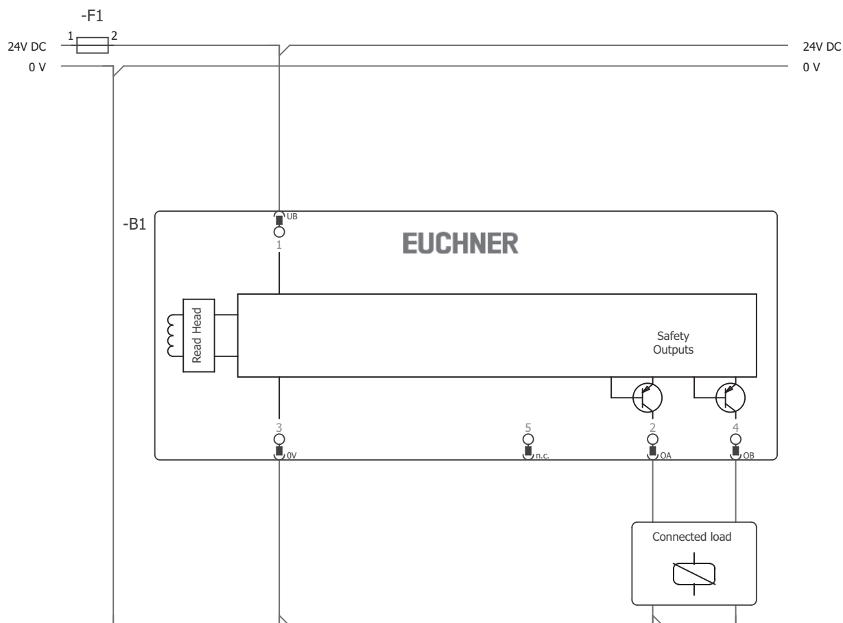
Bild 2: Anschlussbeispiel CES-AP-...
