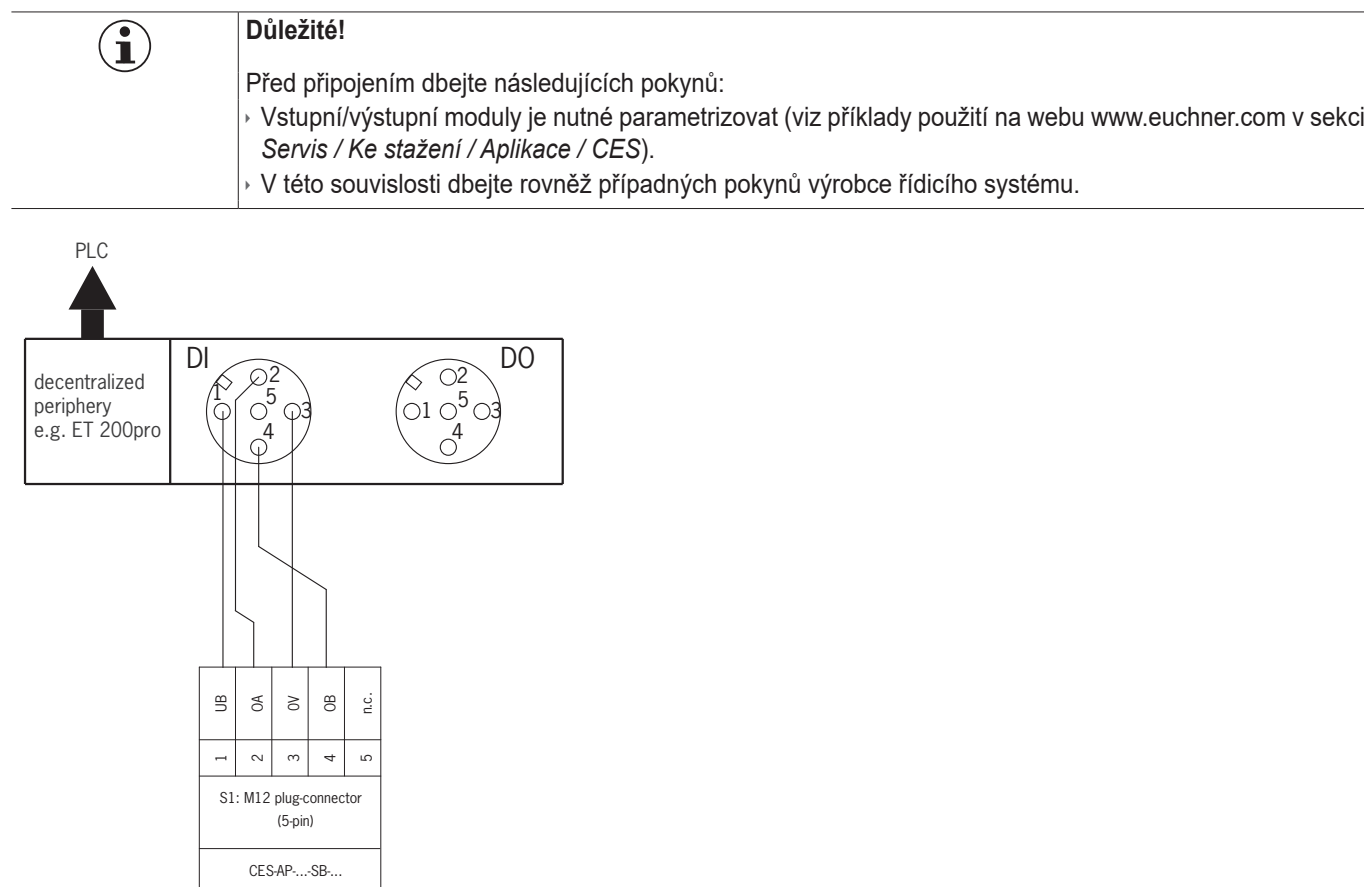
Obr. 3: Příklad připojení: Provedení pro připojení k decentralizovaným periferním systémům
