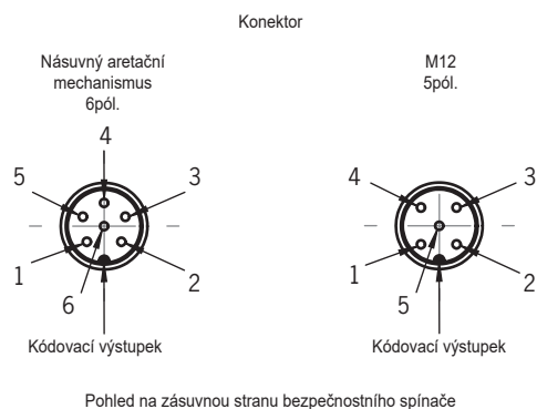
Obr. 1: Obsazení konektoru bezpečnostního spínače CES-AP-C.2
