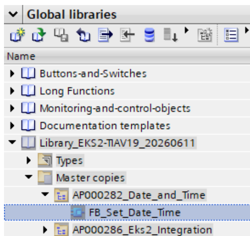
Bild 5: Geöffnete Bibliothek
