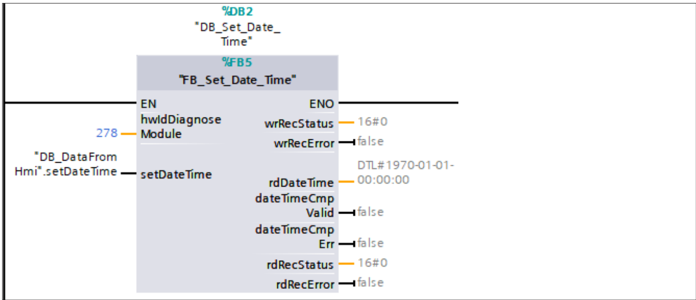
Bild 6: Parametrierter Funktionsbaustein
